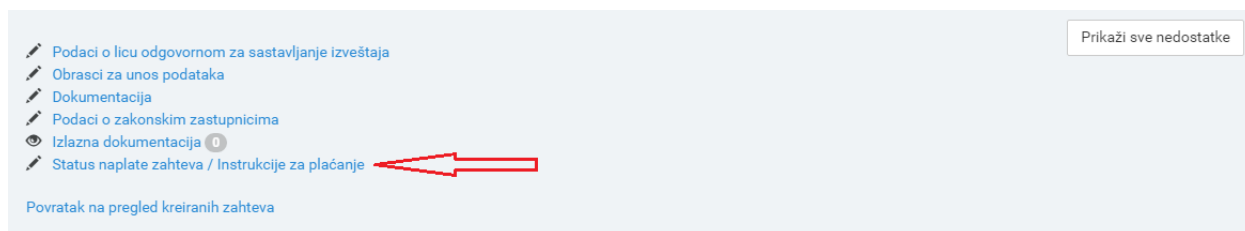
Slika 1. Obrada zahteva
