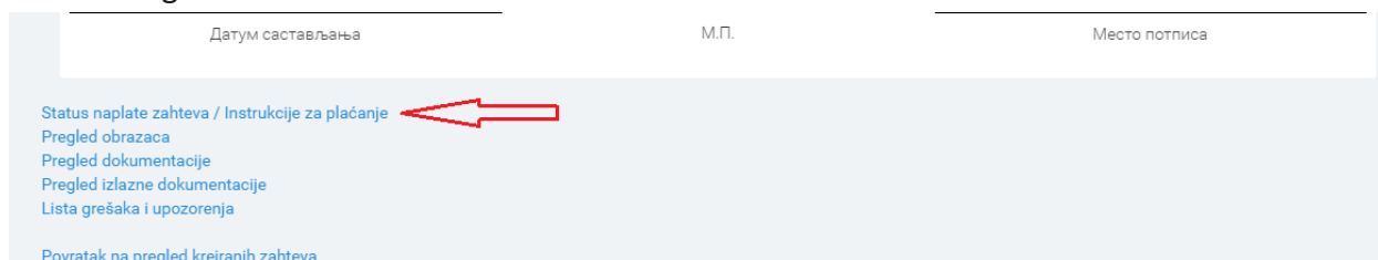
Slika 2. Pregled zahteva
