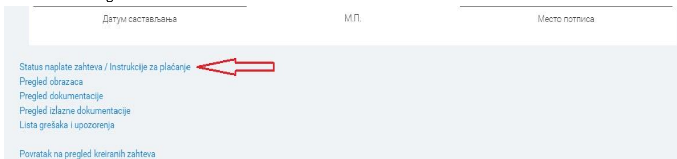
Slika 2. Pregled zahteva
